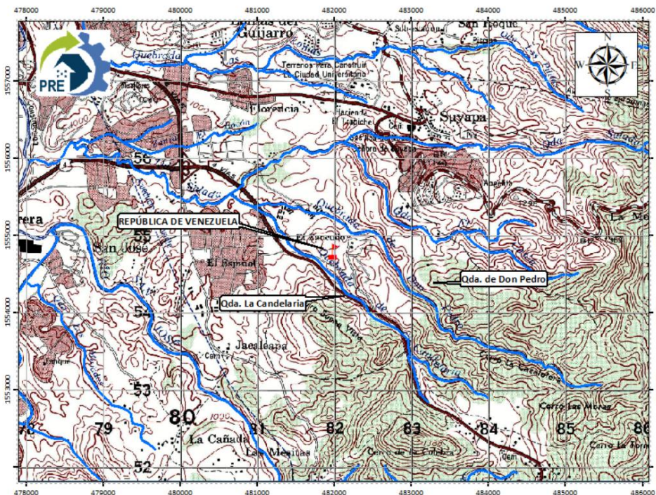
Ilustración 8. Hidrografía del subproyecto
