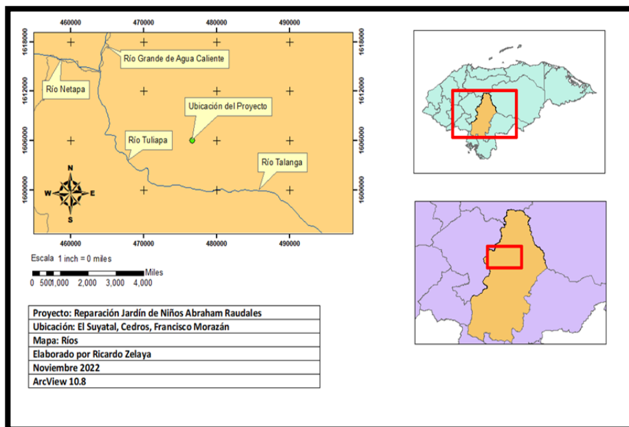
Ilustración 10. Hidrografía regional.
